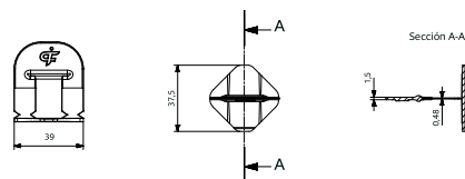
Calzo de cerámica 0,5mm
