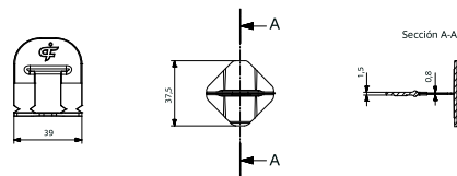
Calzo de cerámica 1mm
